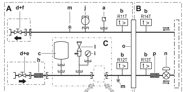
Схема трубопроводов: Модуль гидравлики
