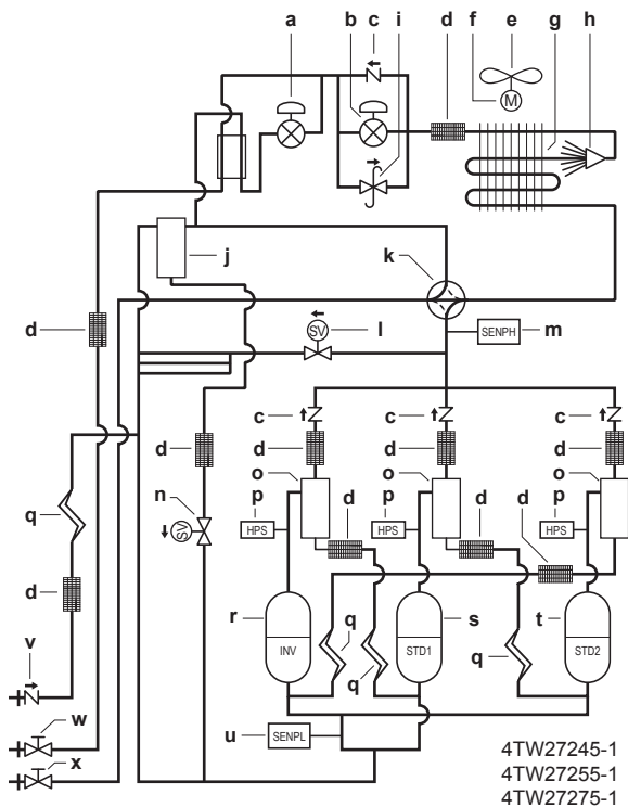
Схема трубопроводов: Наружный модуль
