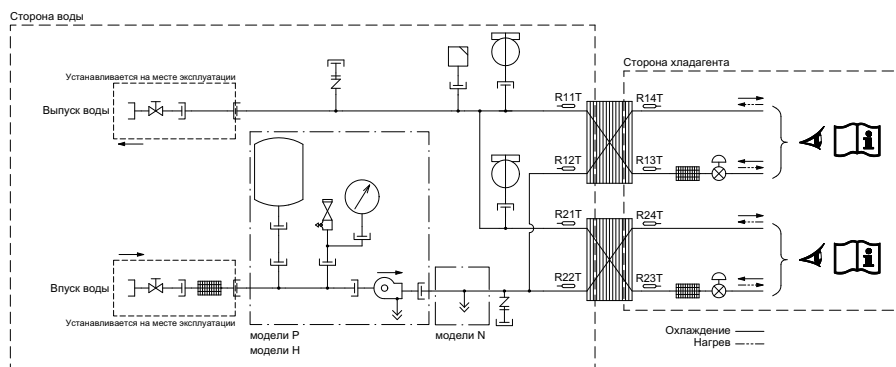
Сочетание небольшого инверторного чиллера и наружного модуля
