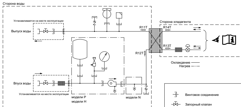
Сочетание небольшого инверторного чиллера и наружного модуля
