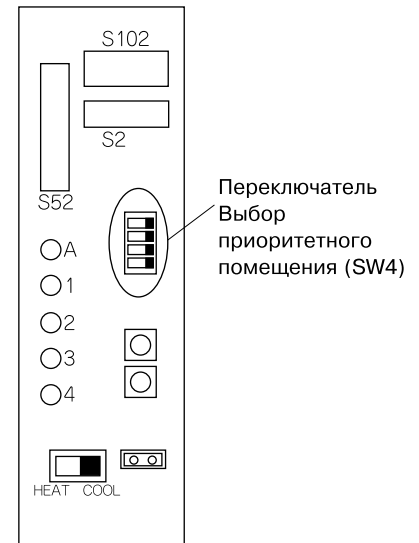
Сервисная Р-плата
