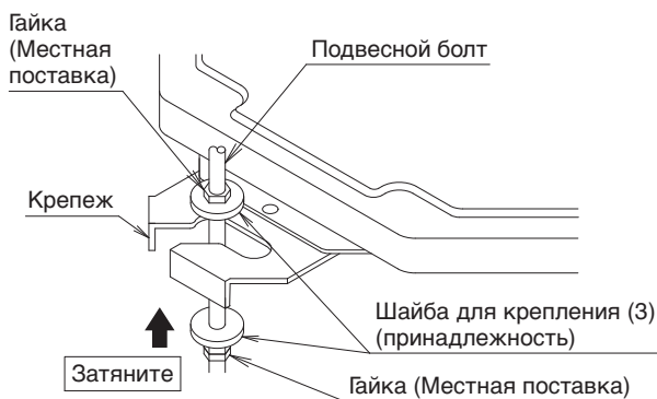
Для фиксирования крепления Рис.15
