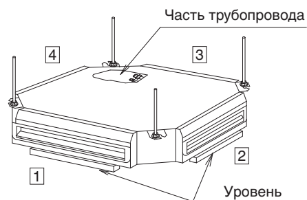
Необходимо обеспечить расположение на одном уровне Рис.18
