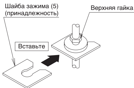
Способ фиксирования шайбы Рис.16
