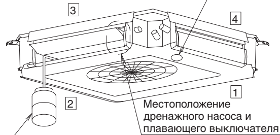
(Как вылить воду) Рис. 34
