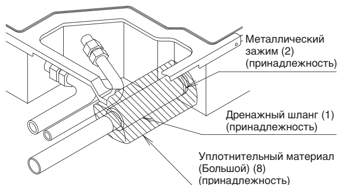
Рис. 27 (Трубопровод, направленный вправо)
