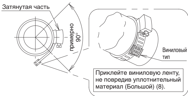
Рис. 32-2 (Раздел А - А Рис. 31)
