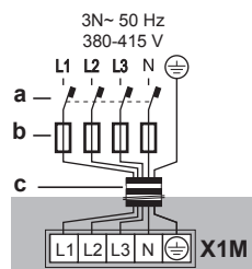
a Предохранитель утечки тока на землю b Плавкий предохранитель c Кабель электропитания
