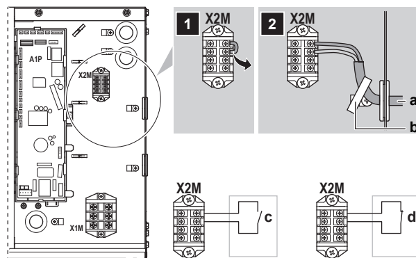
а Контакт для передачи сигнала с дренажного насоса б Кабельная стяжка в Неисправность дренажного насоса: Если контакт размыкается, тепловой насос останавливается и подает сигнал о сбое. Подробнее см. раздел "11.3.1 Коды сбоя: общее представление" на стр. 47. г Нормальная работа дренажного насоса: Если контакт замыкается, тепловой насос возобновляет работу в обычном режиме.
