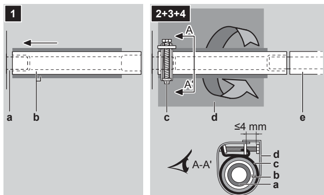
а Соединение сливного трубопровода (с блоком) б Сливной шланг (принадлежность) в Металлический зажим (принадлежность) г Уплотнительная подушка (принадлежность) д Сливной трубопровод (приобретается на месте)
