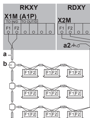
a Изолированный + экранированный кабель (двужильный) (без полярности) a2 Заземление экрана b Клемменная колодка (приобретается по месту установки)
