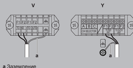
a Заземление
