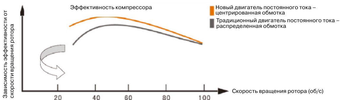
Центрированная обмотка
