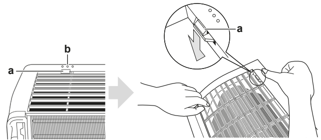
a Верхний крючок b Значок с 3 окружностями
